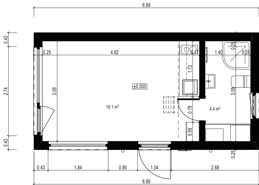
1. STĀVA PLĀNS
