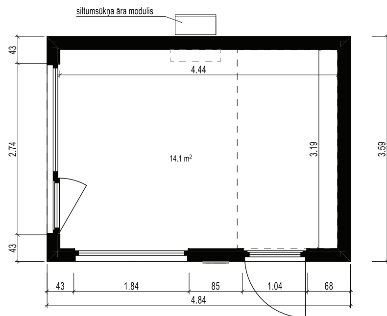
1. STĀVA PLĀNS
