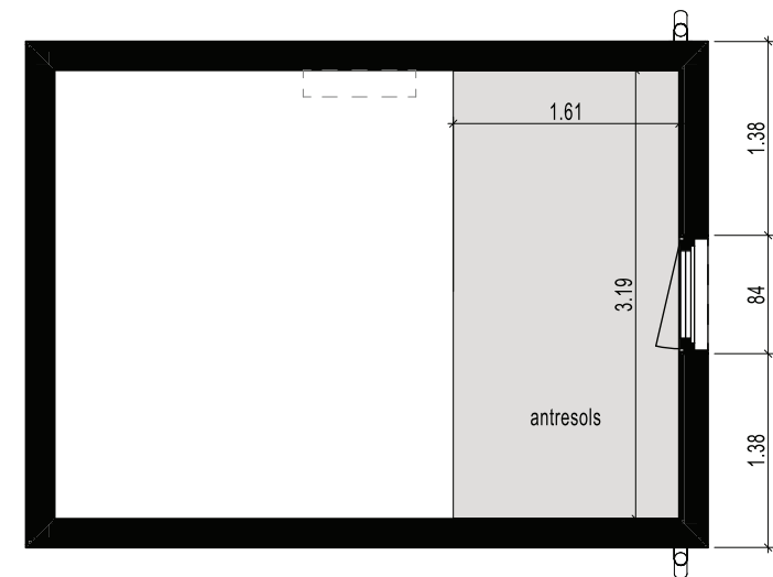
ANTRESOLA PLĀNS
